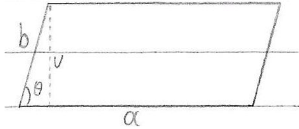
Figure 14: Πλάγιο Παραλληλόγραμμο
