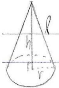
Figure 21: Στοιχεία Κώνου
