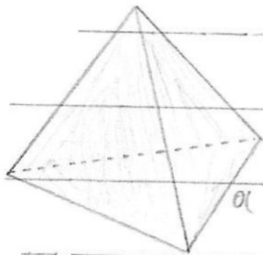
Figure 18: Στοιχεία Τετραέδρου
