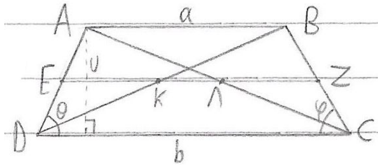
Figure 16: Τραπέζιο
