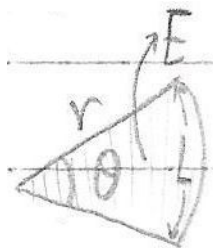
Figure 24: Τόξο κύκλου
