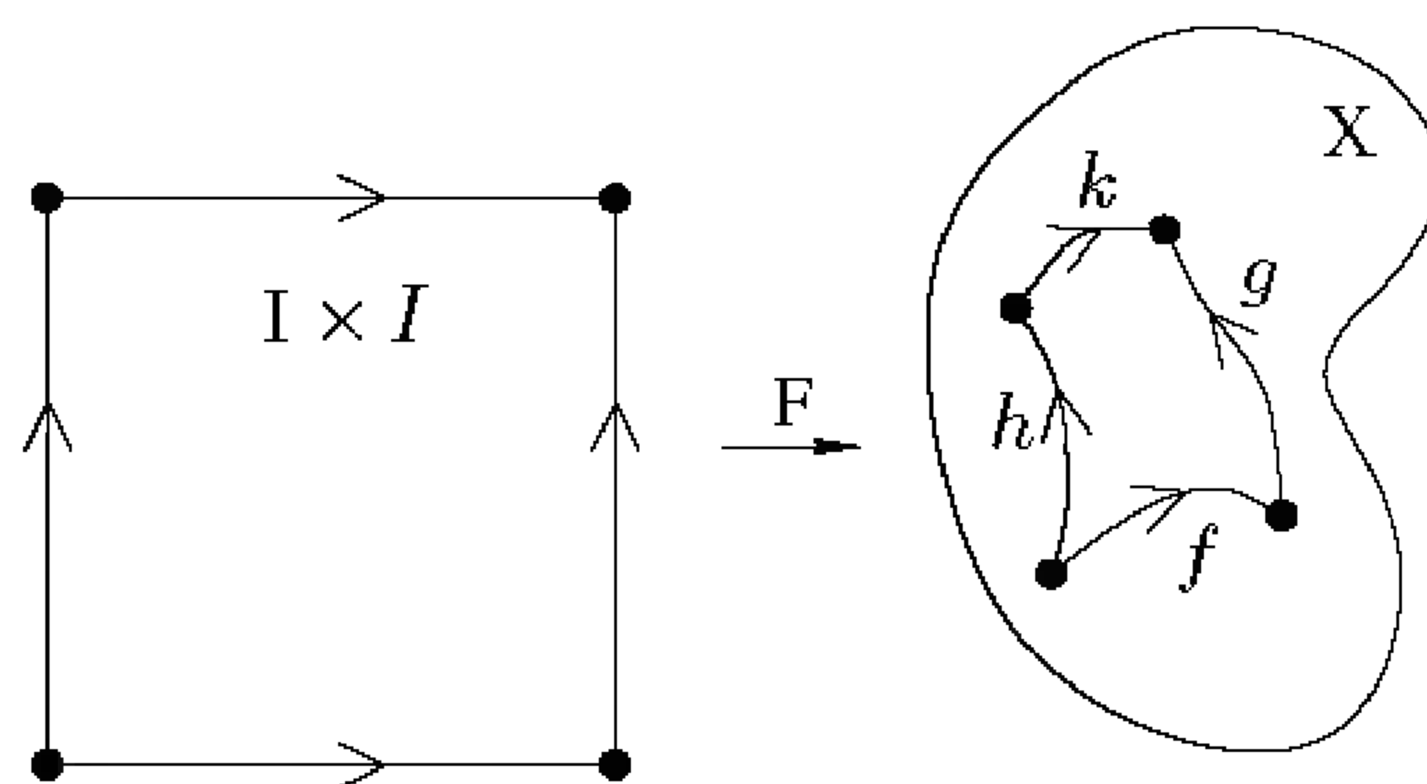
FIGURE 7.7. The map of Lemma 7.12.
