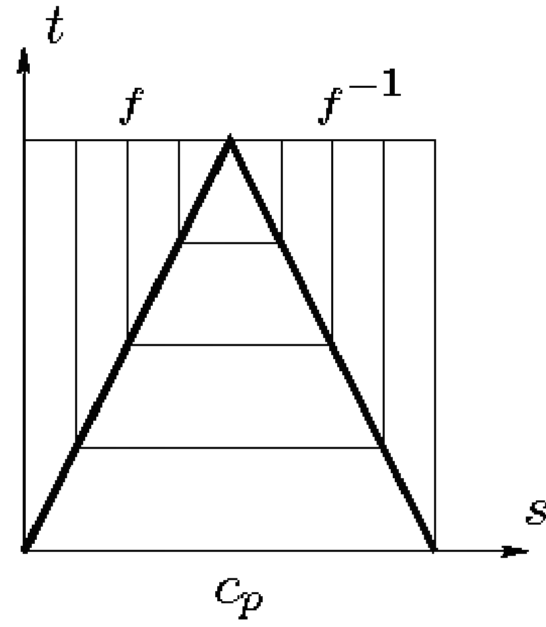
FIGURE 7.5. c_p \sim f \cdot f^{-1} .
