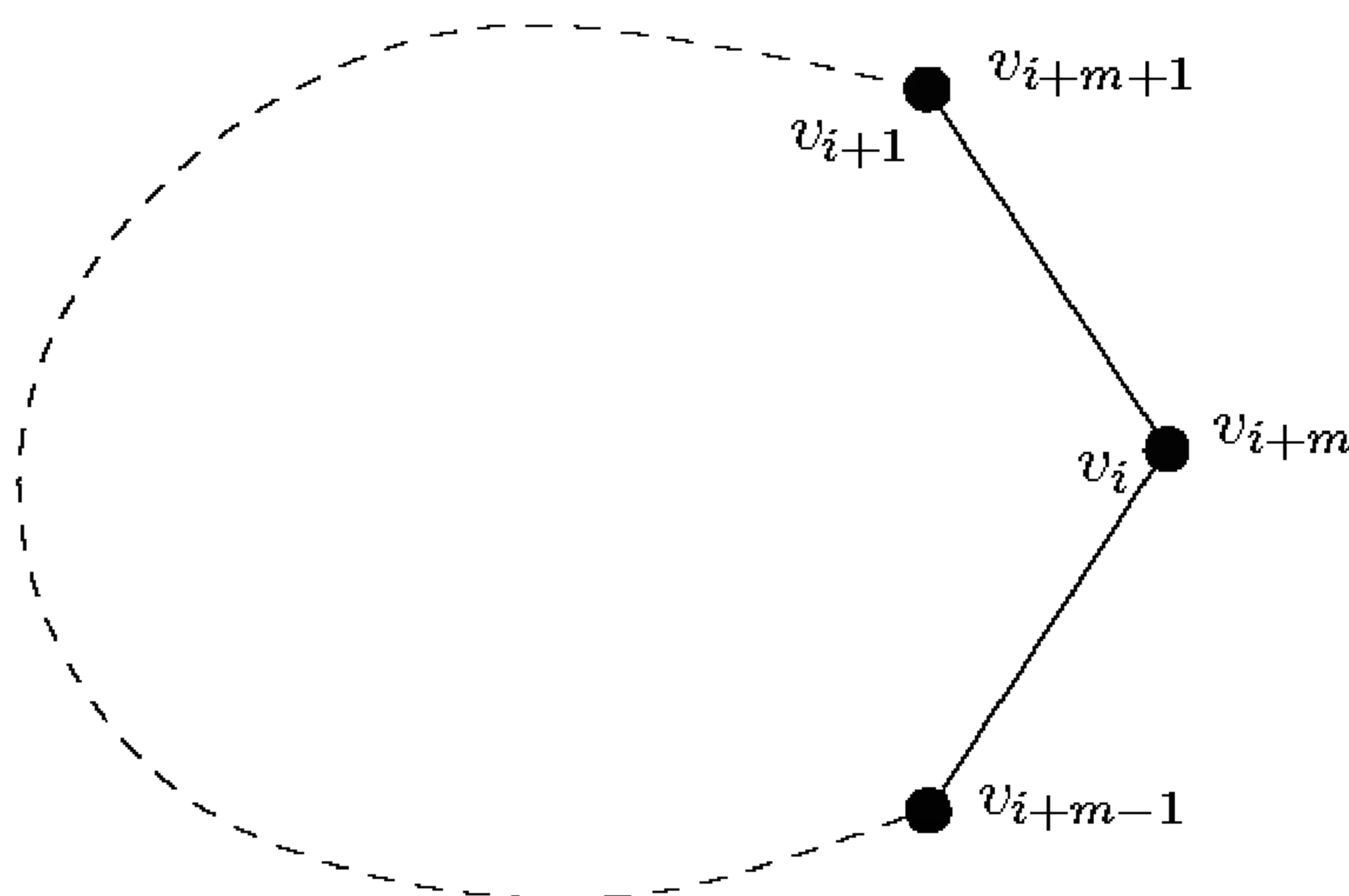
FIGURE 6.1. Periodic edge path.
