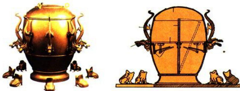
地动仪的复原模型和震动示意图
