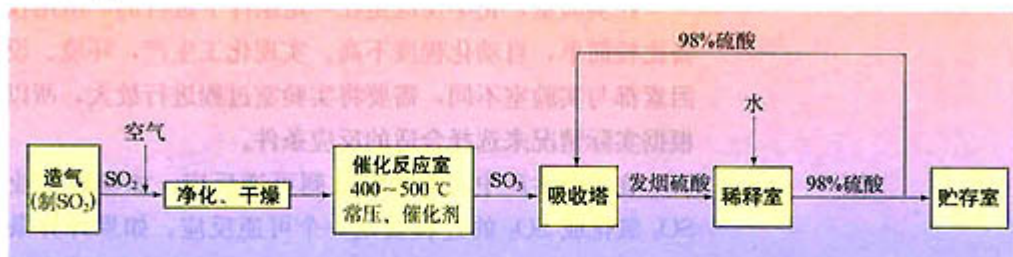
图 1-2 硫酸工业流程
