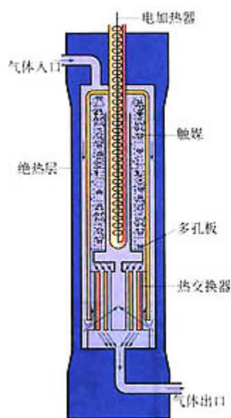
图 1-9 合成塔内部构造示意图 合成塔主要由接触室和热交换器两部分构成；热交换器使合成氨和氨冷凝放出的热量来加热原料气体
