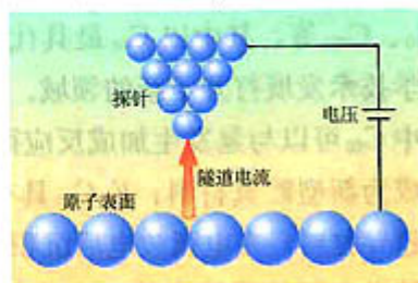
图 3-15 扫描隧道显微镜工作原理示意图
