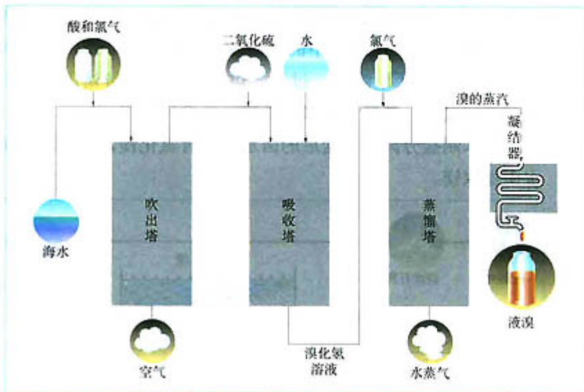
图 2-13 海水提溴吹出法流程
