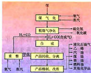
图 2-19 煤间接液化典型流程
