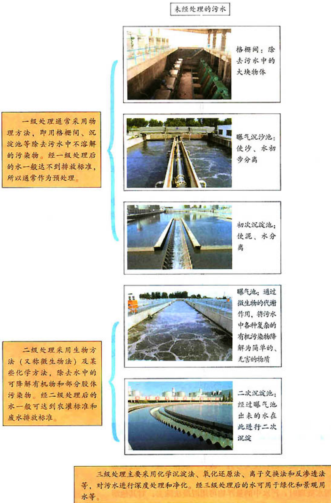
图 2-2 污水处理流程示意图
