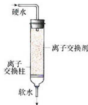
图 2-1 离子交换法软化水示意图
