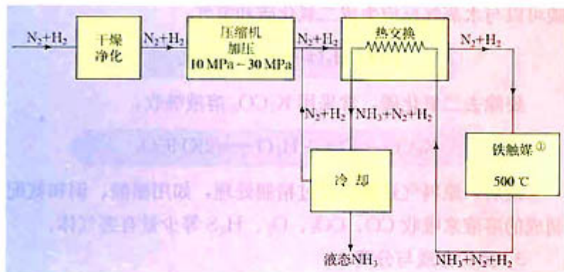
图 1-7 合成氨生产简易流程图示意图
