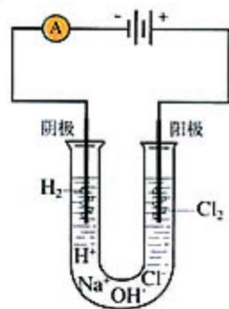
图 2-9 电解饱和食盐水实验装置
