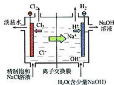
图 2-11 离子交换膜法电解原理示意图
