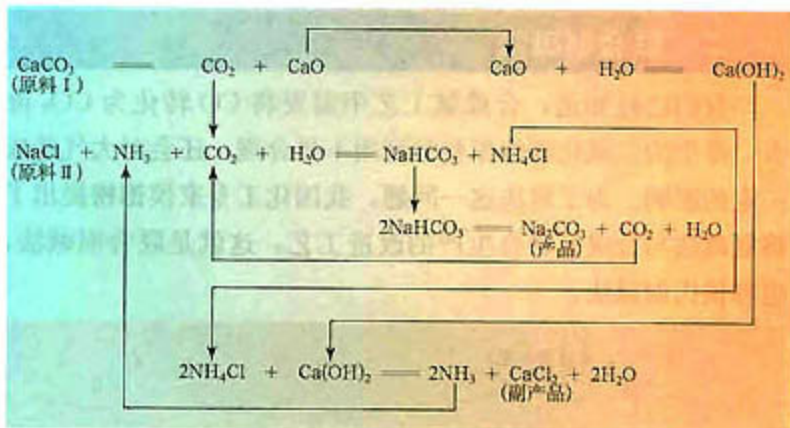
图 1-11 氨碱法生产原理示意图
