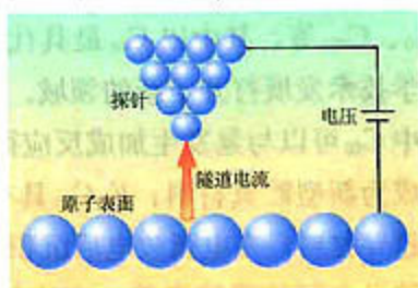
图 3-15 扫描隧道显微镜工作原理示意图
