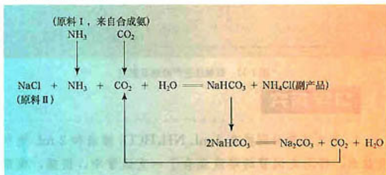
图 1-12 联合制碱法生产原理示意图
