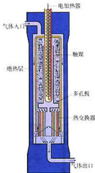
图 1-9 合成塔内部构造示意图
