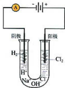
图 2-9 电解饱和食盐水实验装置
