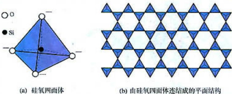
图 3-2 硅氧四面体结构
