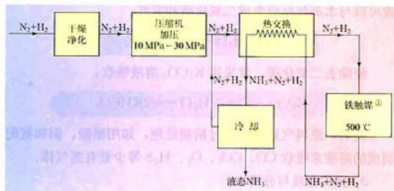
图 1-7 合成氨生产简易流程图
