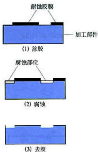
图 3-28 化学蚀刻原理示意图
