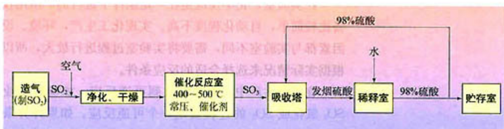
图 1-2 硫酸工业流程
