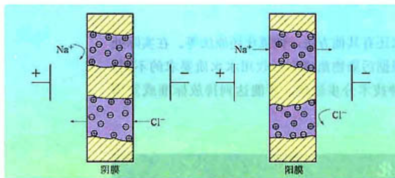
图 2-5 离子交换膜选择透过性示意图
