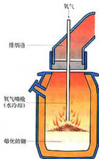
图 3-19 氧气顶吹转炉炼钢示意图
