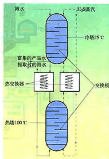
图2-15 硫化氢—水双温交换流程
