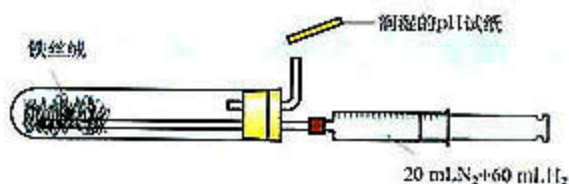
图 1-5 合成氨的实验装置
