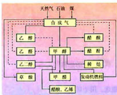
图 2-20 一碳化工产品合成途径
