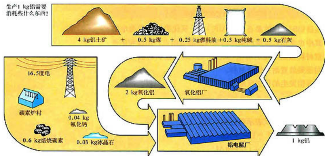
图 3-22 与生产 1 kg 铝相关连的消耗
