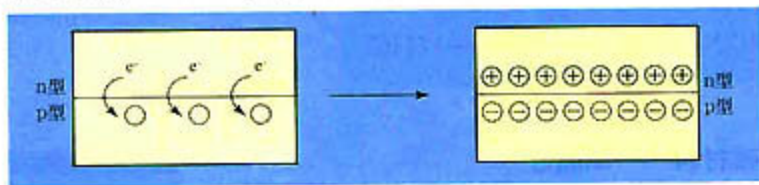
图3-11 p-n结中电子的转移示意图
