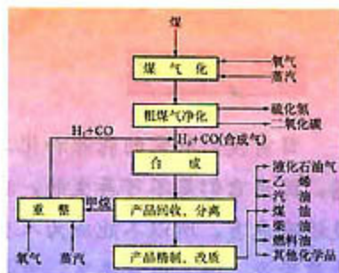
图 2-19 煤间接液化典型流程
