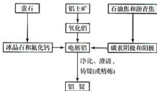
图 3-20 铝的生产流程示意图
