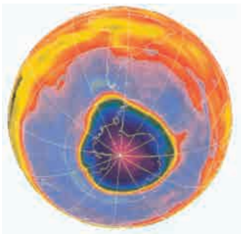
在南极上空,紫色和粉红色区域表明臭氧层的严重衰竭状态
