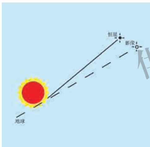
光线在太阳引力场中的弯曲
