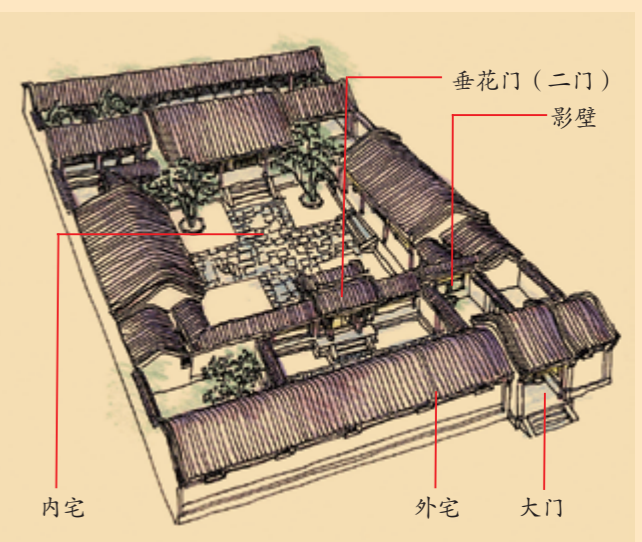
四合院示意图 (北京)
