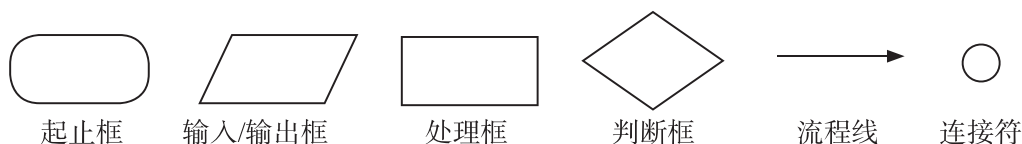
图2.1.1 流程图符号
