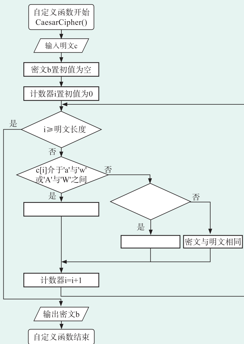
图3.4.1 恺撒加密算法流程图
