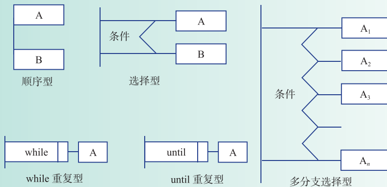
图4.1.4 PAD图
