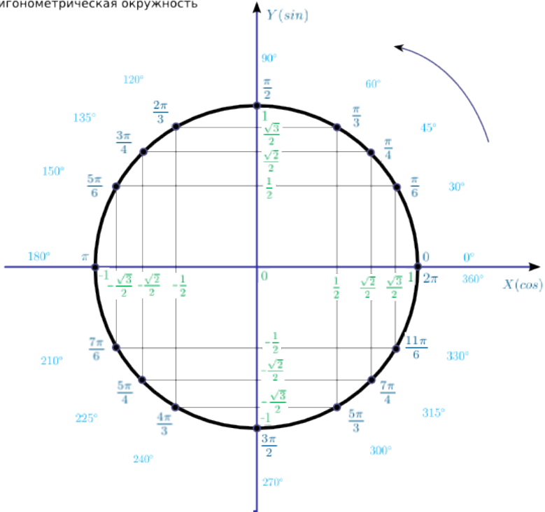
Тригонометрическая окружность
